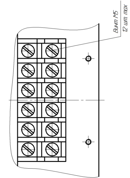
Рисунок А.7 – Варианты исполнения вторичных выводов (крышка защитная условно не показана)
