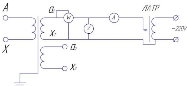
Рисунок 5 – Схема проведения испытания для трансформаторов, предназначенных для измерения линейных напряжений, с двумя вторичными обмотками
