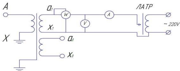
Рисунок 1 – Схема проведения испытания для трансформаторов, предназначенных для измерения фазных напряжений, с двумя вторичными обмотками: с одной основной и одной дополнительной
