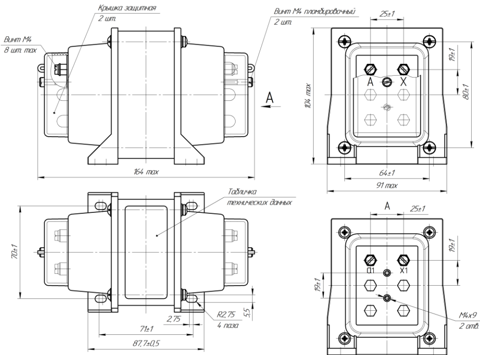
Рисунок А.1 – Габаритные, установочные, присоединительные размеры трансформаторов НОП-НТ3-1
