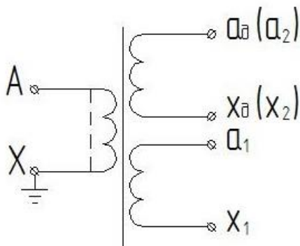
Рисунок Б.2 – Схема электрическая принципиальная трансформаторов, предназначенных для измерения фазных напряжений, с двумя вторичными обмотками
