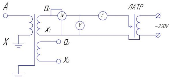
Рисунок 2 – Схема проведения испытания для трансформаторов, предназначенных для измерения фазных напряжений, с двумя основными вторичными обмотками
