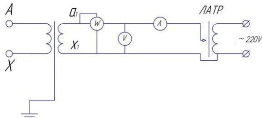
Рисунок 4 – Схема проведения испытания для трансформаторов, предназначенных для измерения линейных напряжений, с одной вторичной обмоткой
