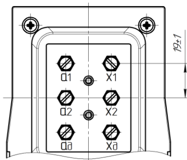
Рисунок А.2 – Габаритные, установочные, присоединительные размеры трансформаторов НОП-НТЗ-1
