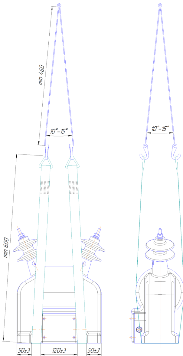
Рисунок Г.1 – Схема строповки трансформаторов ОЛ-НТЗ-0,63/6(10)-IV
