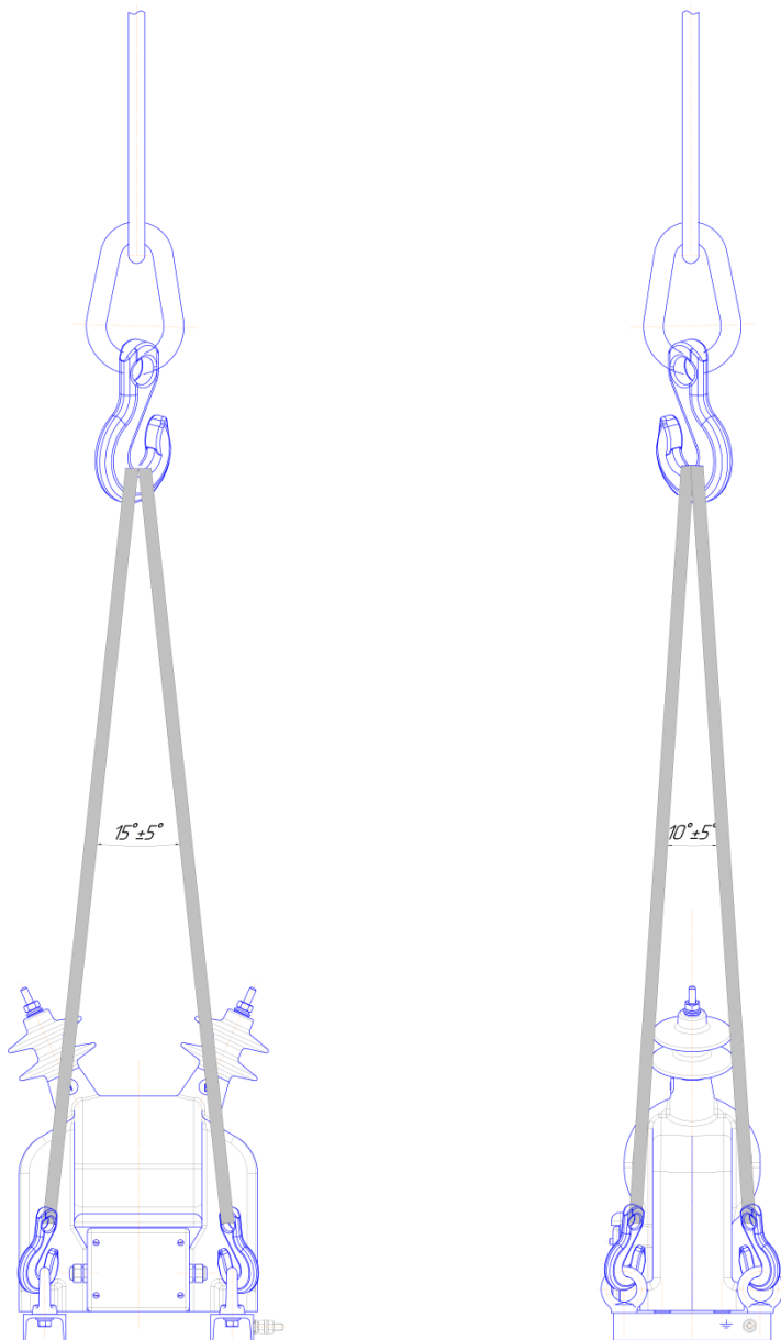
Рисунок Г.2 – Схема строповки трансформаторов ОЛ-НТЗ-0,63/6(10)-IV-01
