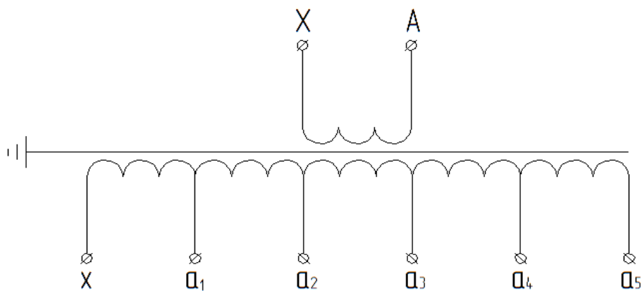
Рисунок В.1 - Схема электрическая принципиальная ОЛ-НТЗ-0,63/6(10)-IV
