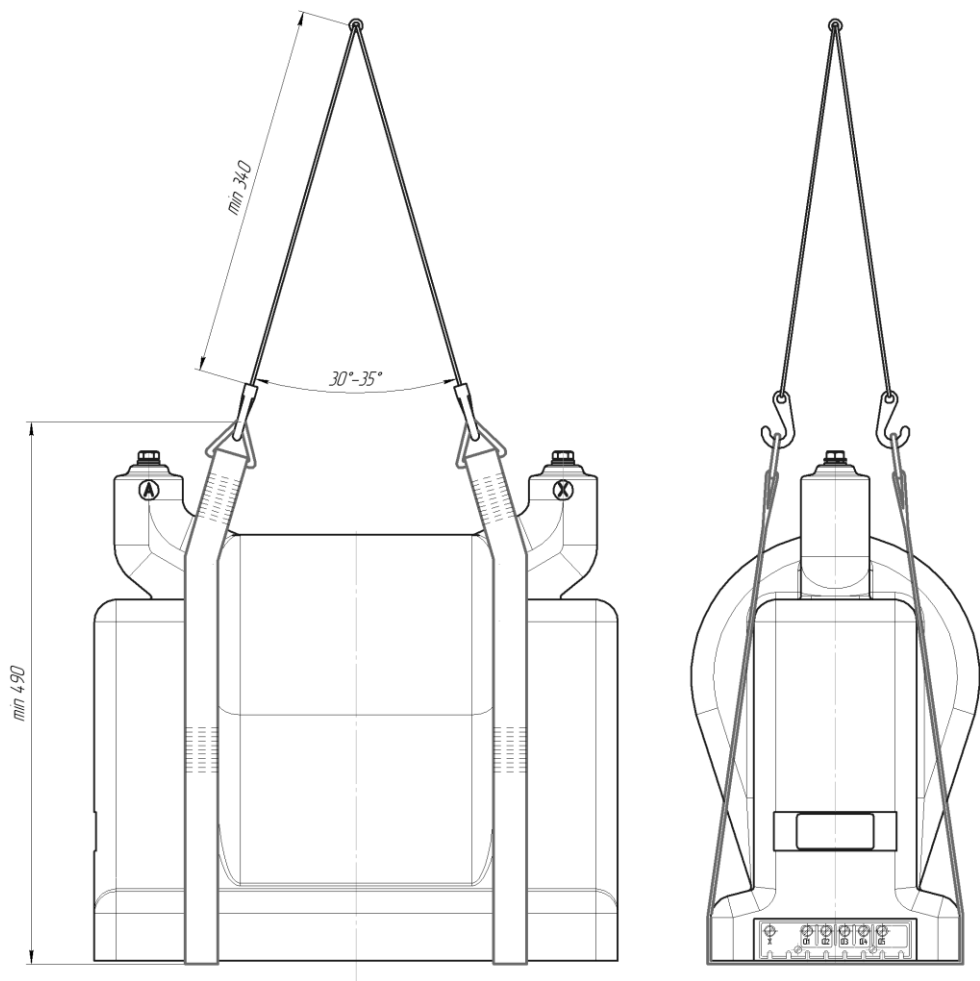
Рисунок В.1 – Схема строповки трансформаторов ОЛС-НТЗ-10/6(10,20)
