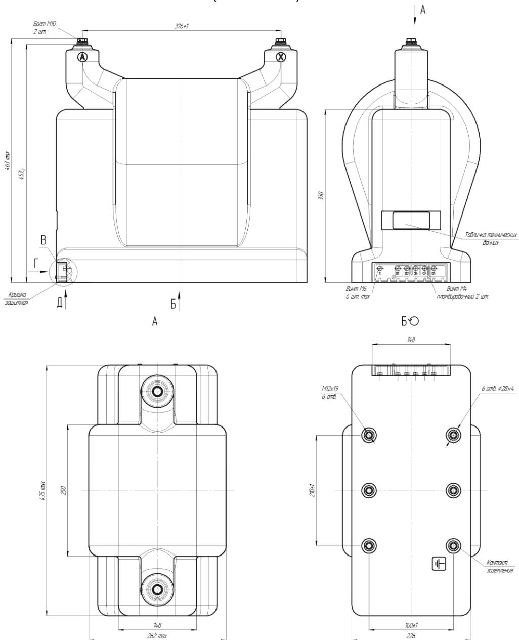
Рисунок А.1 – Габаритные установочные, присоединительные размеры и масса трансформаторов ОЛС-НТЗ-10/6(10,20)
