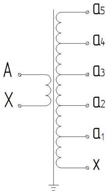
Рисунок Б.1 - Схема электрическая принципиальная ОЛС-НТЗ-10/6(10,20)
