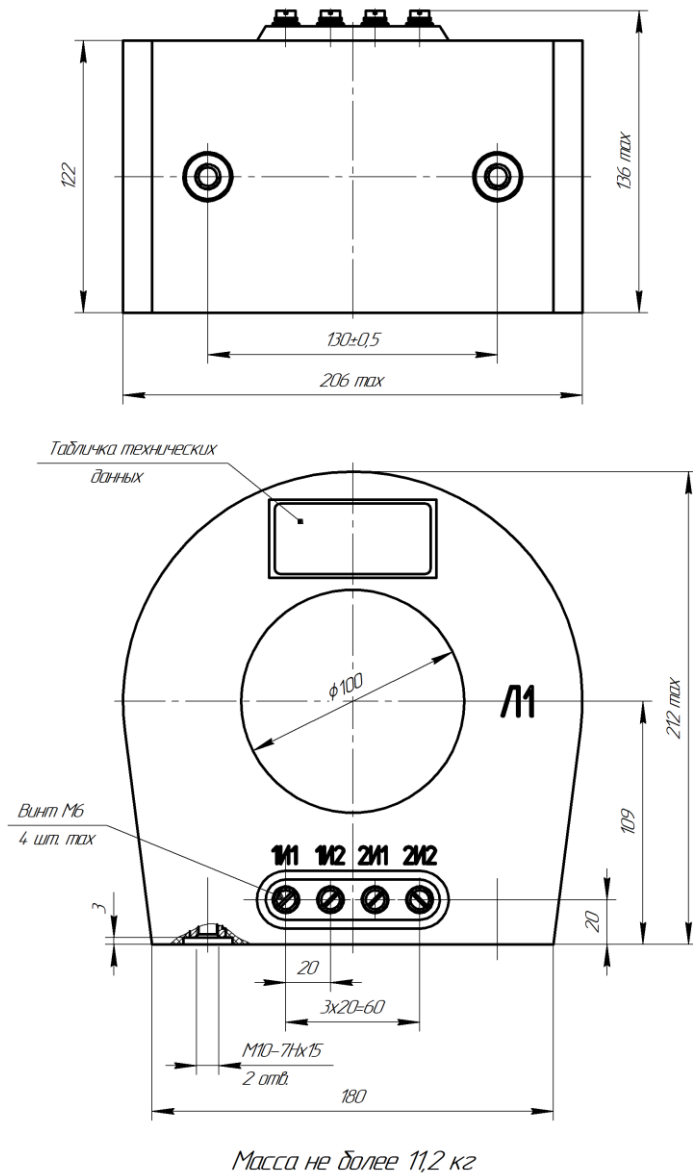
Рисунок А.2 – Габаритные, установочные, присоединительные размеры и масса трансформаторов ТЗЛК-НТЗ-0,66-100-01
