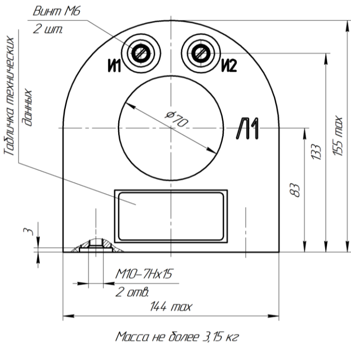
Рисунок А.1 – Габаритные, установочные и присоединительные размеры трансформаторов ТЗЛК-НТЗ-0,66-70 МЗ
