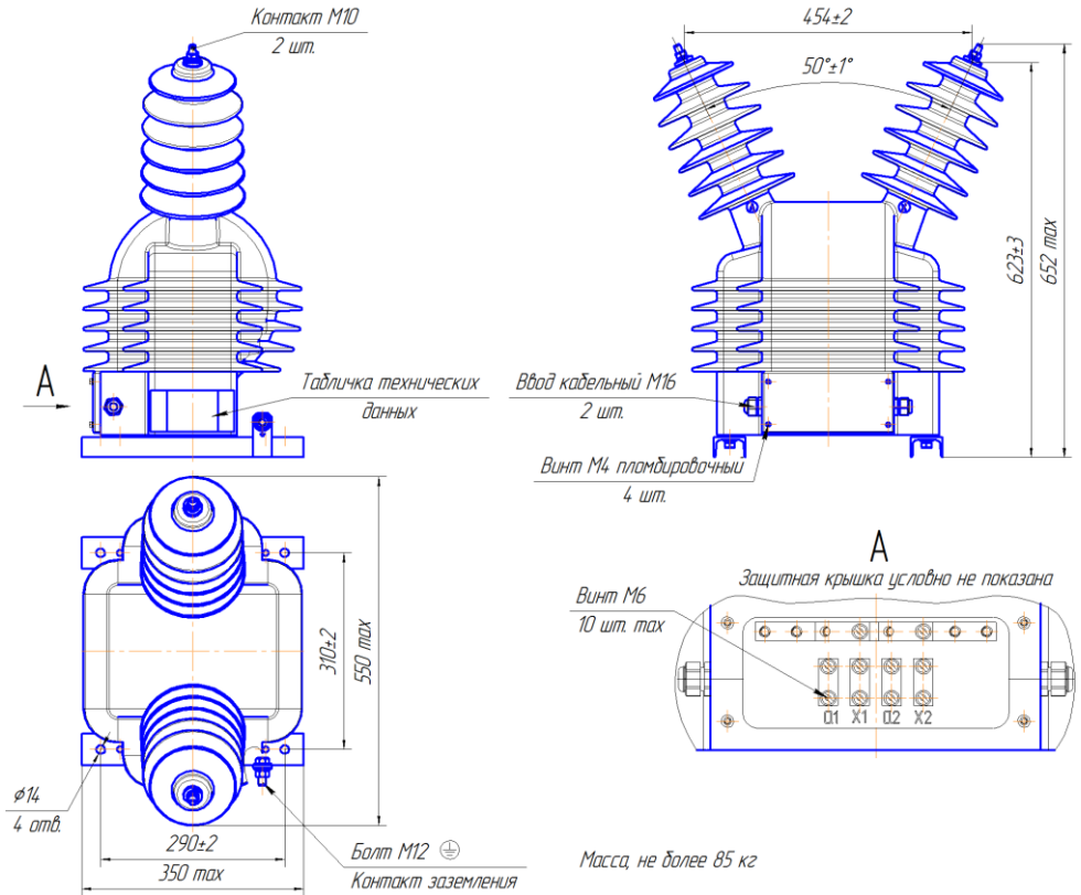
Рисунок Б.1 – Габаритные установочные, присоединительные размеры и масса трансформаторов ОЛ-НТЗ-1,25/35-IV
