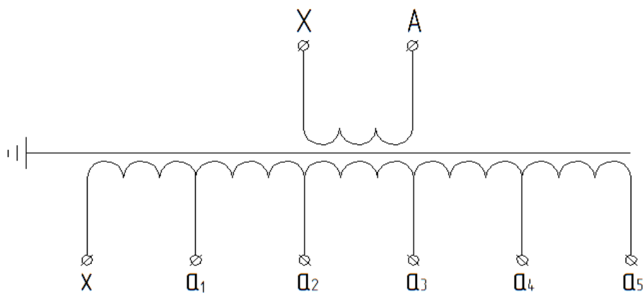
Рисунок В.1 - Схема электрическая принципиальная ОЛ-НТЗ-1,25/35-IV
