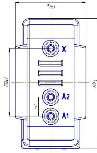
Рисунок А.1 – Габаритные, установочные, присоединительные размеры и масса трансформатора НОЛ-НТЗ-20
