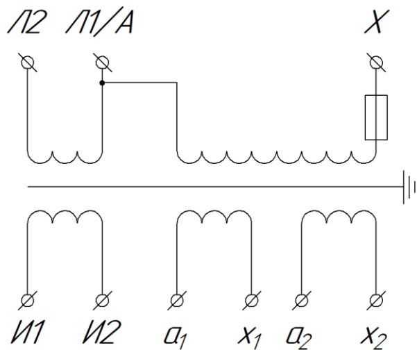
Рисунок Б.1 – Схема электрическая принципиальная для трансформаторов НТОЛП-НТЗ-6(10)-IV
