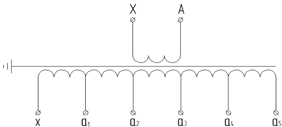
Рисунок В.1 - Схема электрическая принципиальная ОЛ-НТЗ-1,25/6(10)(-01)-IV
