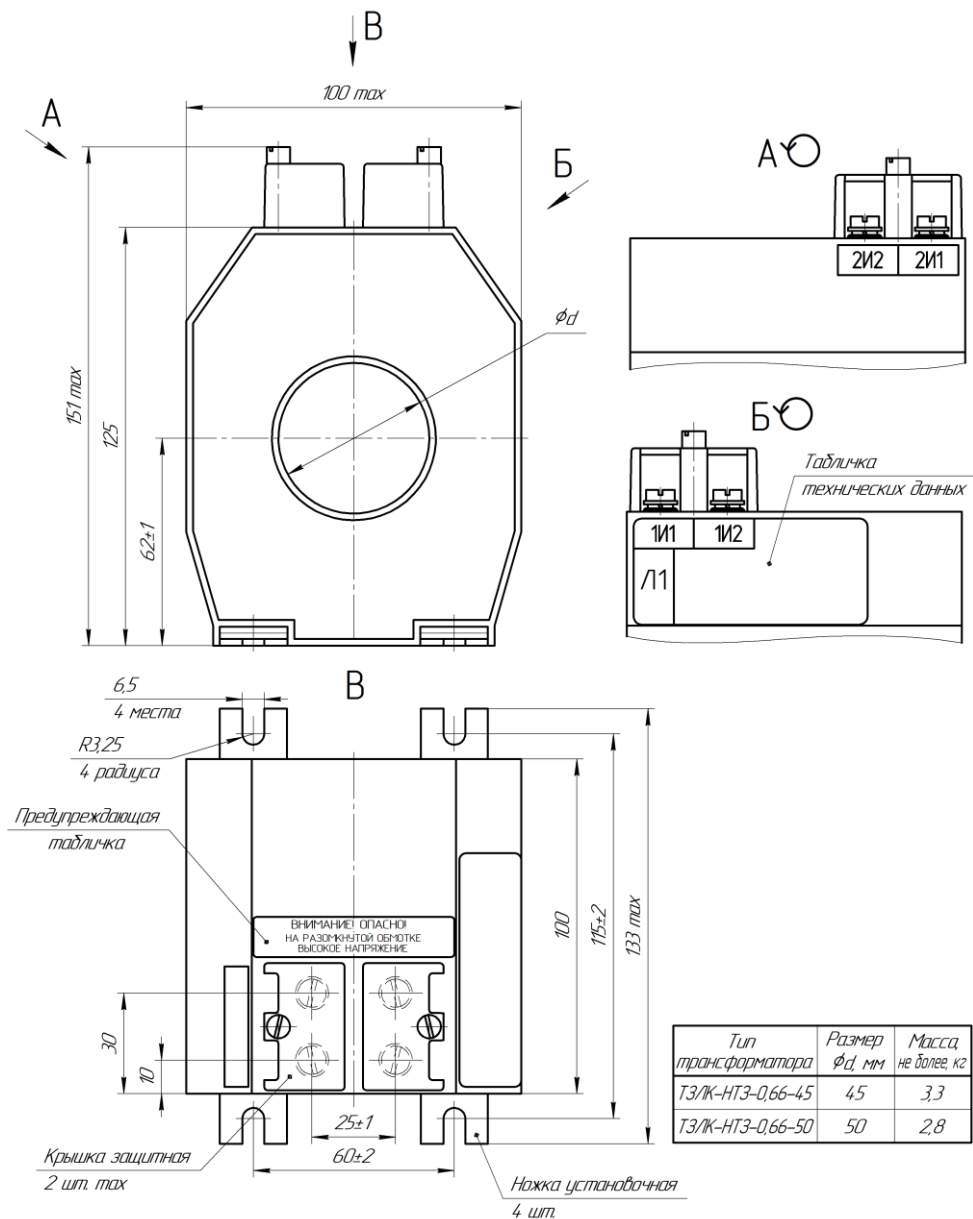
Рисунок А.1 – Габаритные, установочные, присоединительные размеры и масса трансформаторов ТЗЛК-НТЗ-0,66-45(-50)
