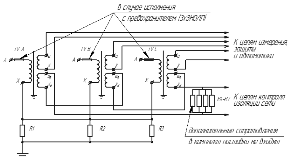
Рисунок Б.1 – Схема электрическая принципиальная трёхфазной группы трансформаторов напряжения 3хЗНОЛ(П)-НТЗ-6(10)
