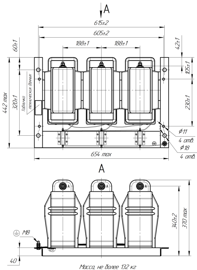
Рисунок А.7 – Габаритные, установочные, присоединительные размеры и масса трехфазных групп 3хЭНОЛП-НТЗ-6(10)-04
