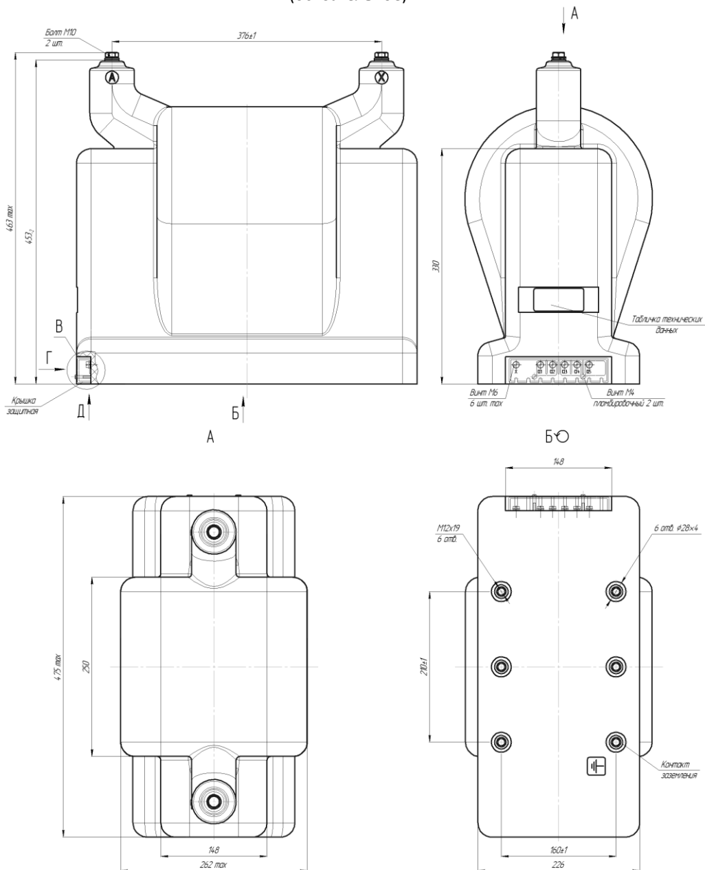
Рисунок А.1 – Габаритные установочные, присоединительные размеры и масса трансформаторов ОЛС-НТЗ-10(13,5)/6 (10,20)
