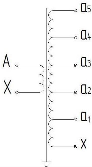
Рисунок Б.1 - Схема электрическая принципиальная ОЛС-НТЗ-10(13,5)/6 (10,20)
