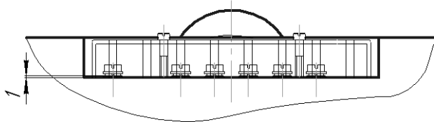
Рисунок А.2 – Исполнение вторичных выводов трансформаторов ОЛС-НТЗ-10(13,5)/6 (10,20)
