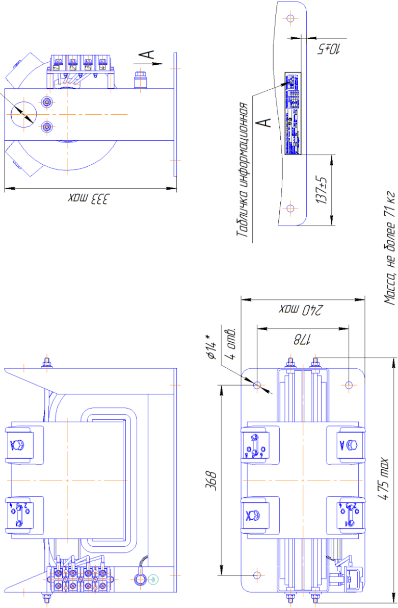
Рисунок А.1 – Габаритные, установочные, присоединительные размеры и масса трансформаторов ОЛС-НТЗ-5,0/6(10)
